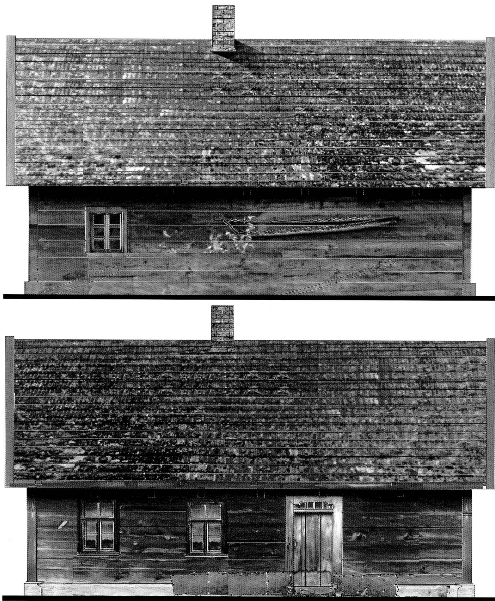
10-13. Rysunki inwentaryzacyjne elewacji domu nr 41. Rys. Aleksandra Bednarska, 2016. Inventory diagrams of the elevation of house no. 41. Drawing: Aleksandra Bednarska, 2016.
